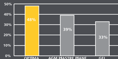
DŁUGOŚĆ CYKLU WOBEC SZYBKości ROZŁADOWANIA W AKUMULATORACH OPTIMA
